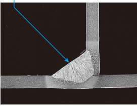
ビード部 溶接断面
